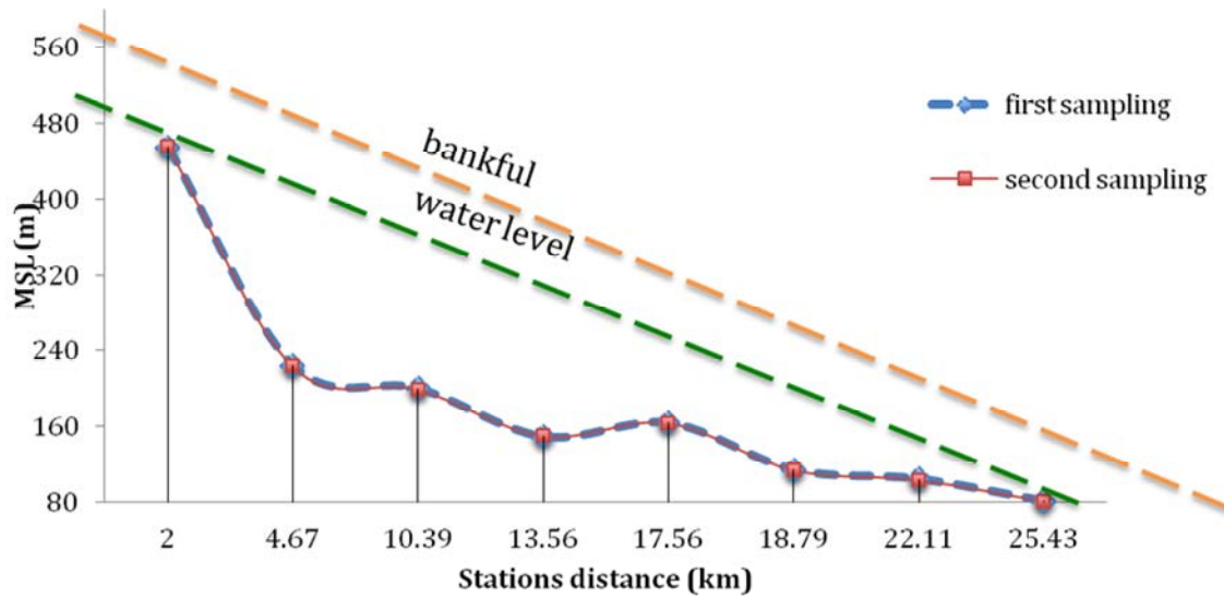
Fig. 2: Longitudinal profile
