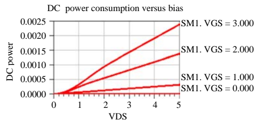
Fig. 4: DC Power-VDS
