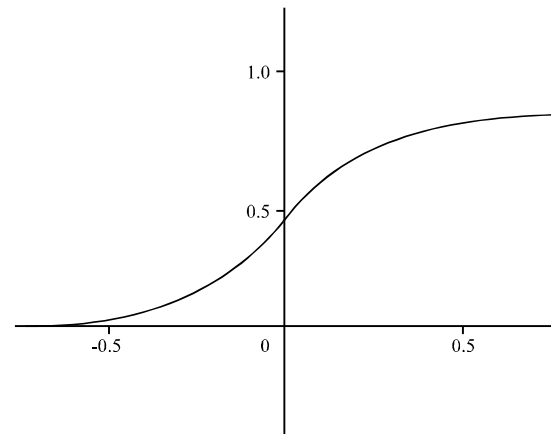
Fig. 2: Sigmoid function
