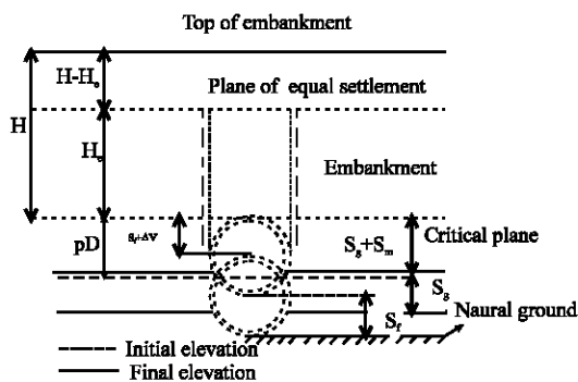
Fig. 2: Rigid conduit
